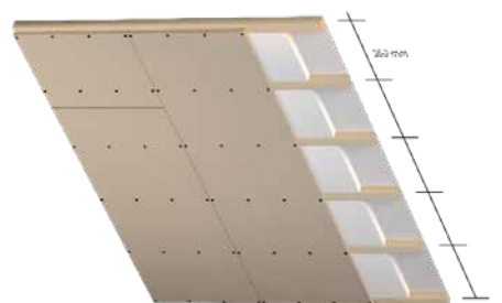
Ansicht Dachschräge
