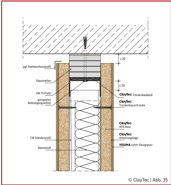
Metallunterkonstruktion Anschluss an Massivdecke, gleitend
