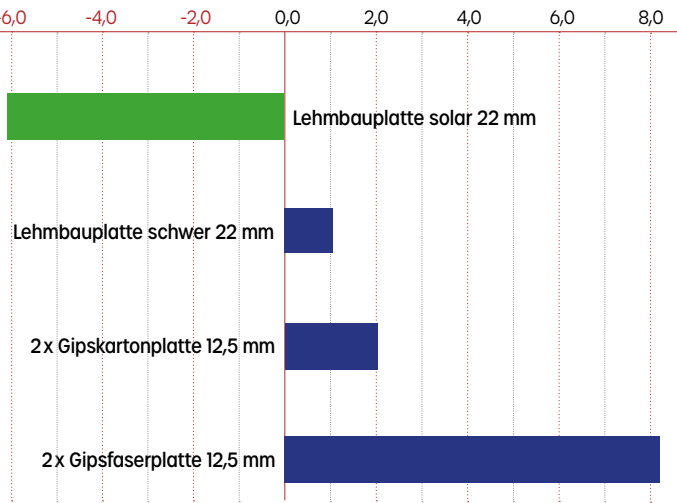
GWP ausgewählter Trockenbauplatten, kg CO 2 Äquiv./m 2
