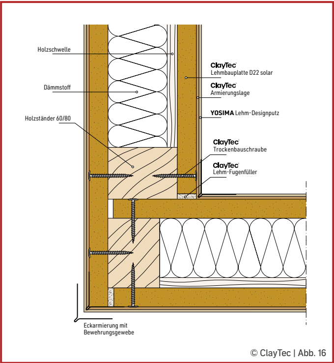
Holzkonstruktion Eckanschluss
