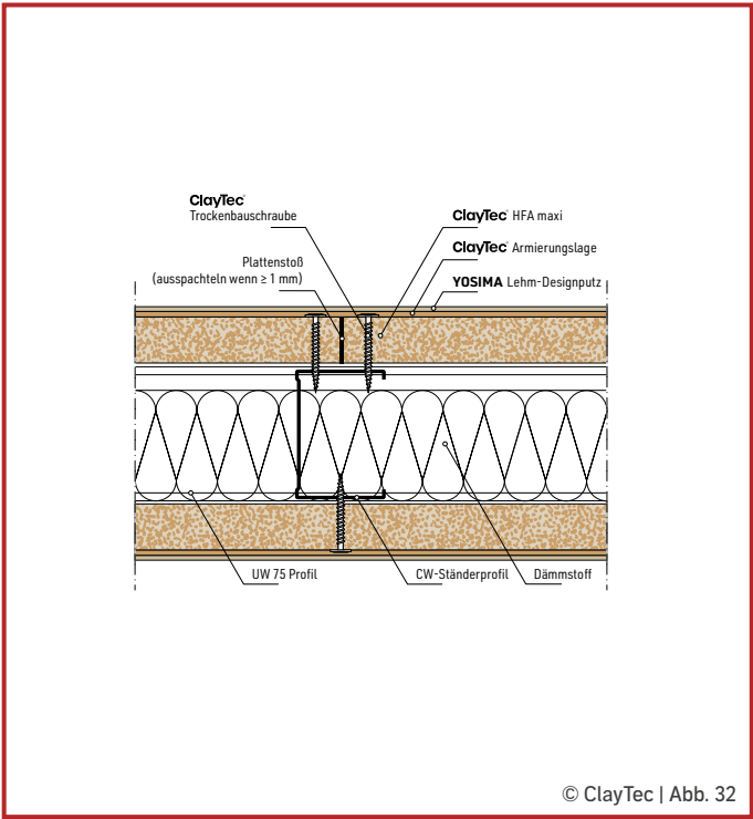
Metallunterkonstruktion Plattenstoß horizontal
