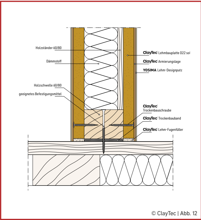
Holzkonstruktion Anschluss an Holzbalkenboden
