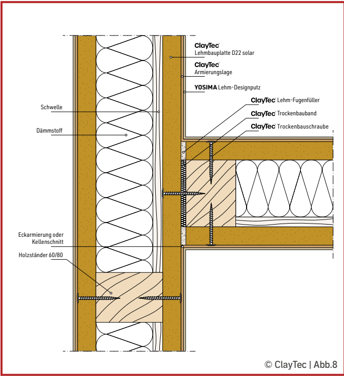
Holzkonstruktion Anschluss an Trockenbauwand
