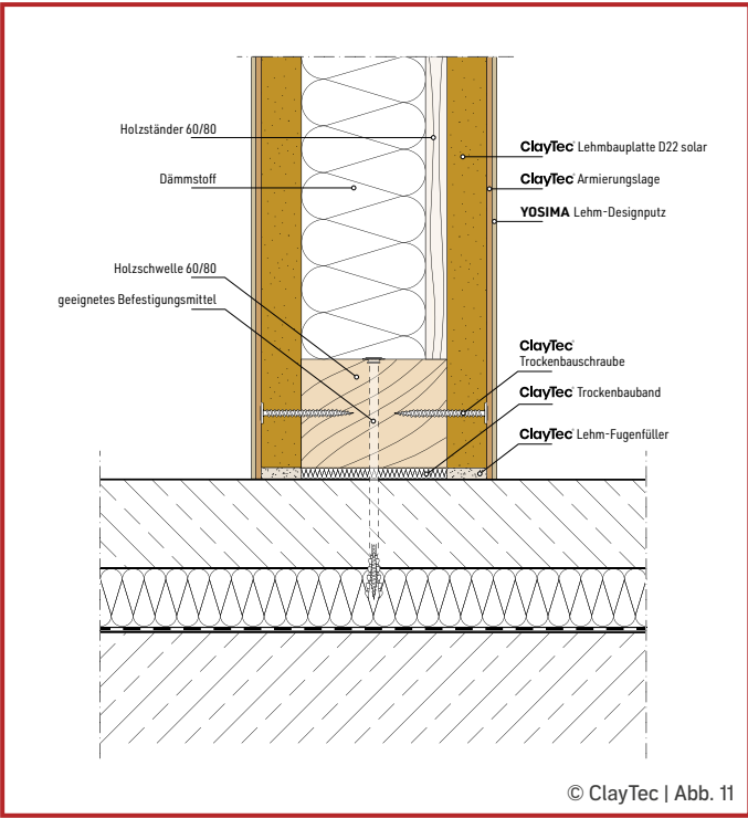
Holzkonstruktion Anschluss an Massivboden
