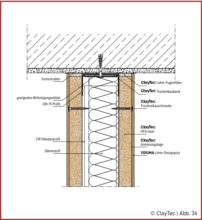
Metallunterkonstruktion Anschluss an Massivdecke
