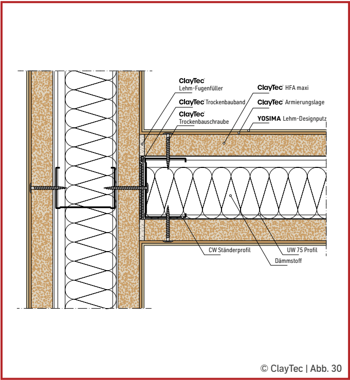
Metallunterkonstruktion Anschluss an Trockenbauwand
