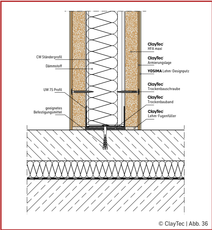
Metallunterkonstruktion Anschluss an Massivboden
