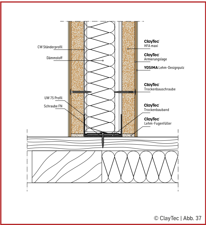
Metallunterkonstruktion Anschluss an Holzbalkenboden
