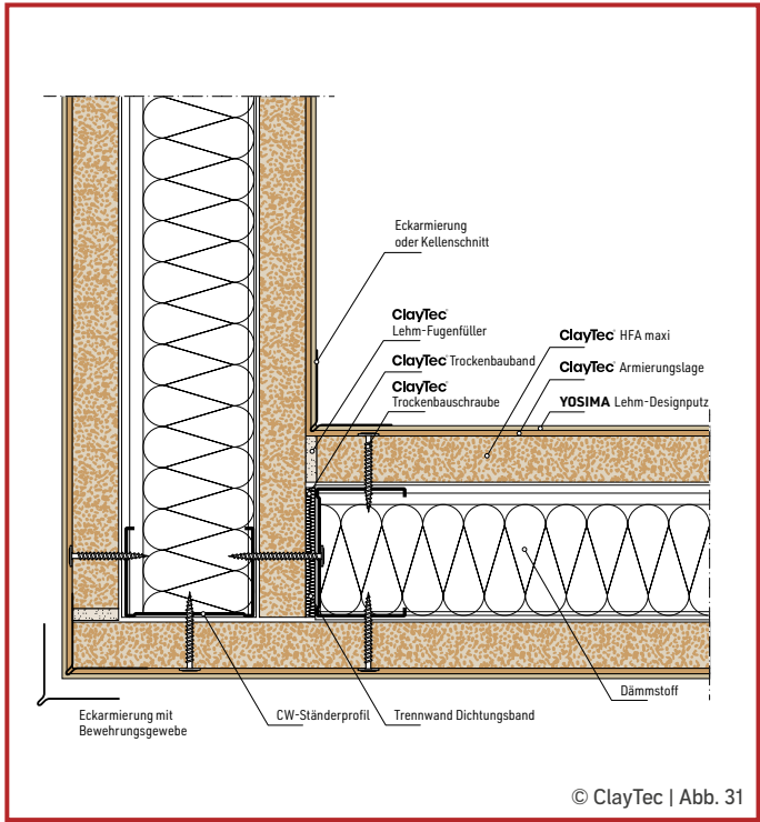
Metallunterkonstruktion Eckanschluss
