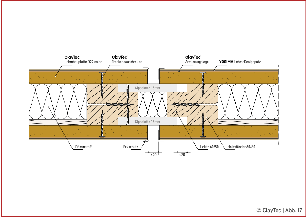
Holzkonstruktion Bewegungsfuge
