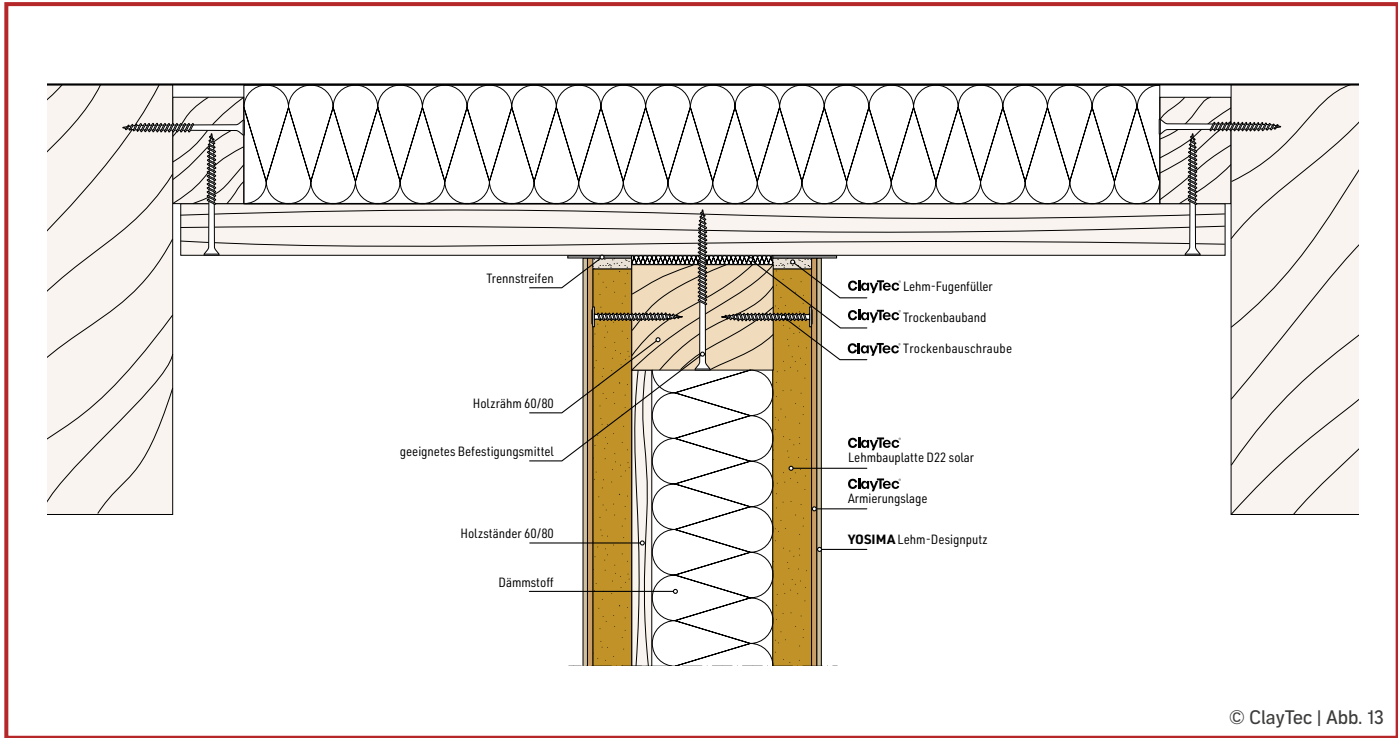
Holzkonstruktion Anschluss an Decke, Holzbalken sichtbar
