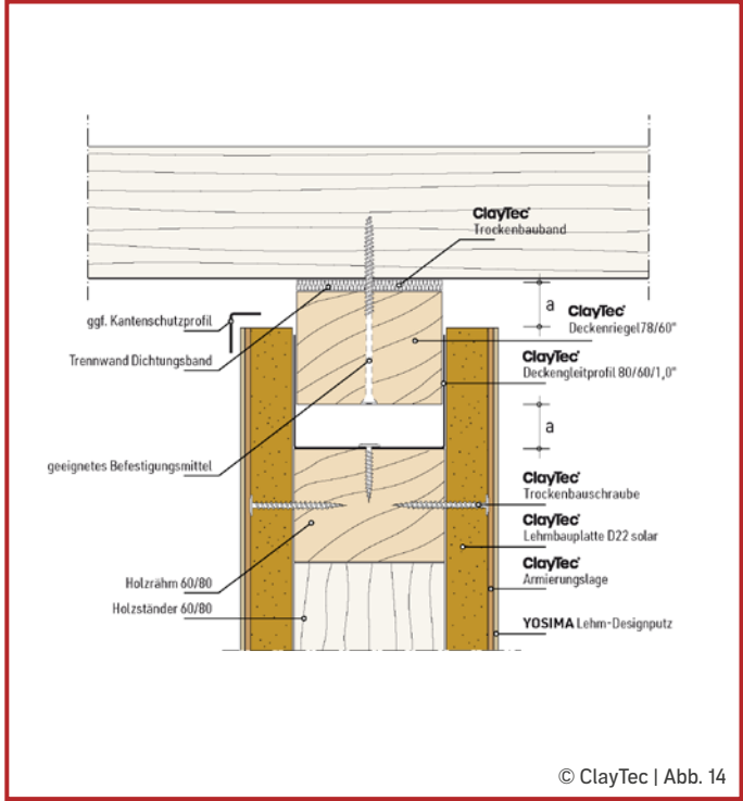
Holzkonstruktion Anschluss an Holzdecke, gleitend
