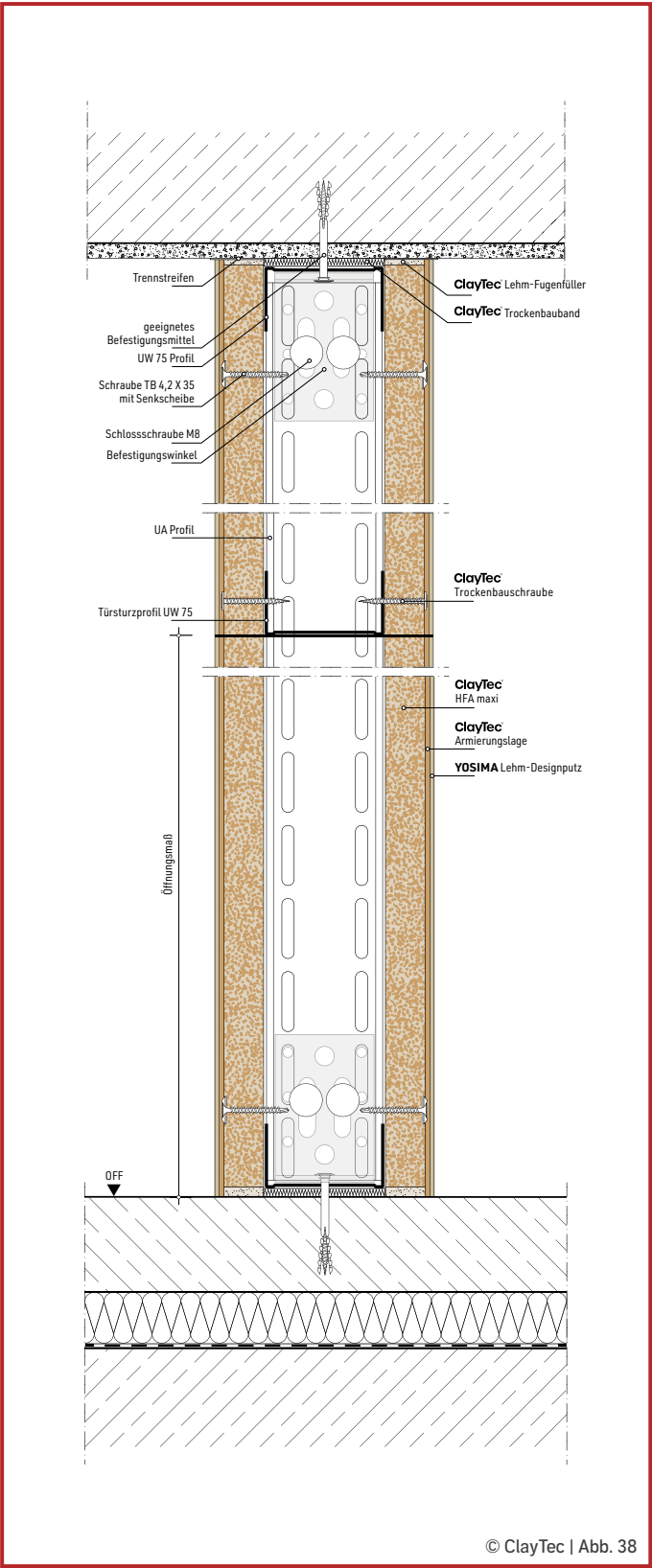
Metallkonstruktion Türöffnung vertikal
