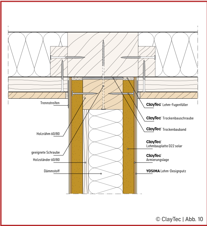
Holzkonstruktion Anschluss an Holzbalkendecke
