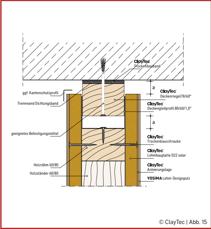
Holzkonstruktion Anschluss an Massivdecke, gleitend
