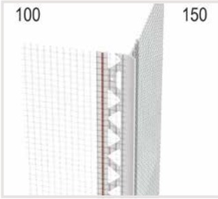
Gewebeeckwinkel mit Abzugskante (100 x 150 mm/3 mm), PROTEKTOR Art.-Nr. 37521
