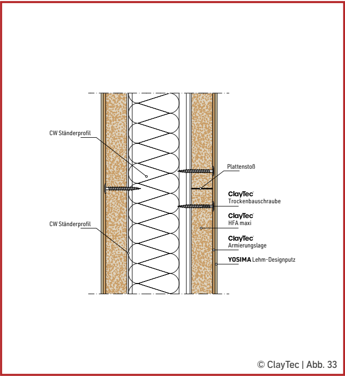
Metallunterkonstruktion Plattenvorstoß vertikal
