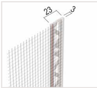
Abschlussprofil mit Gewebe (3 mm) PROTEKTOR Art.-Nr. 3793
