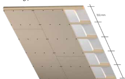
Plaatsing plafond
