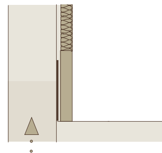
Fußpunkt mit Abdichtung und Schaumglasdämmung
