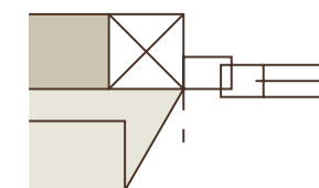
Fensteranschluss \leq 30^\circ
