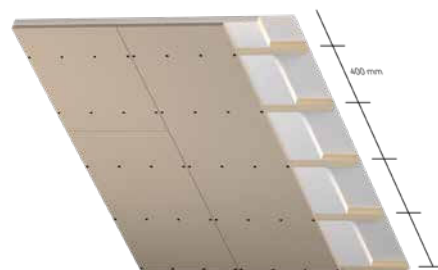
Ansicht Dachschräge
