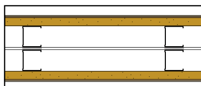
Metallkonstruktion Doppelständerwand
