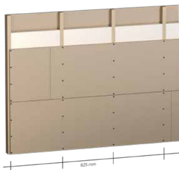
Ansicht Wand
